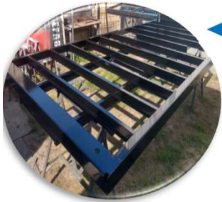
BASES Metálicas, con perímetro de chapas estampadas y teleras de I.P.N
